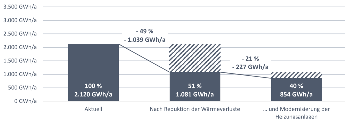
Endenergieverbrauch für Wärme im Haushaltssektor
